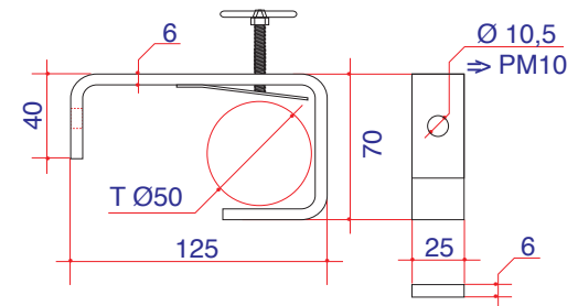
ACL.25.006 Zn ou Preto
