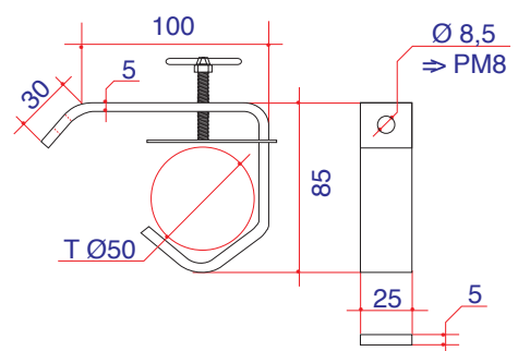
ACL.25.005 Zn ou Preto
