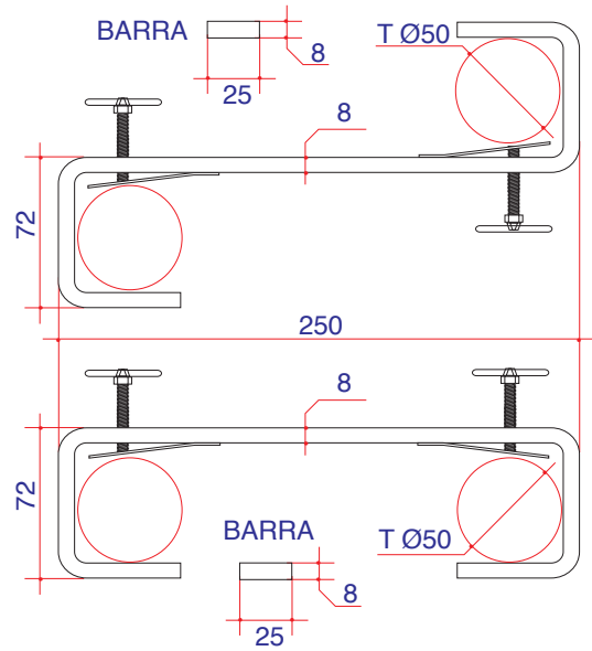
ACL.25.308 Zn (Zincado)
